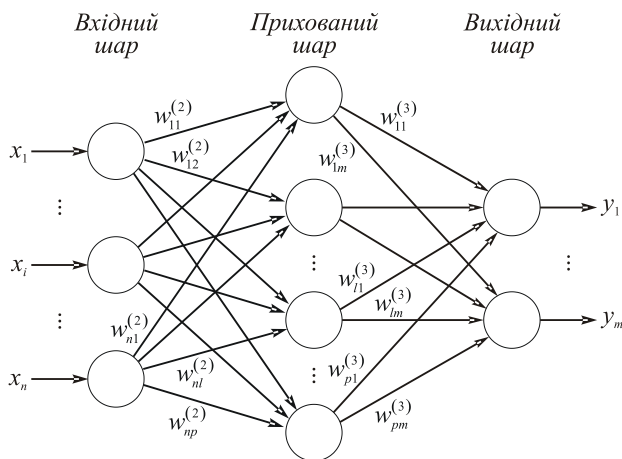
Рис. 3. Структура нейронної мережі типу персептрон
