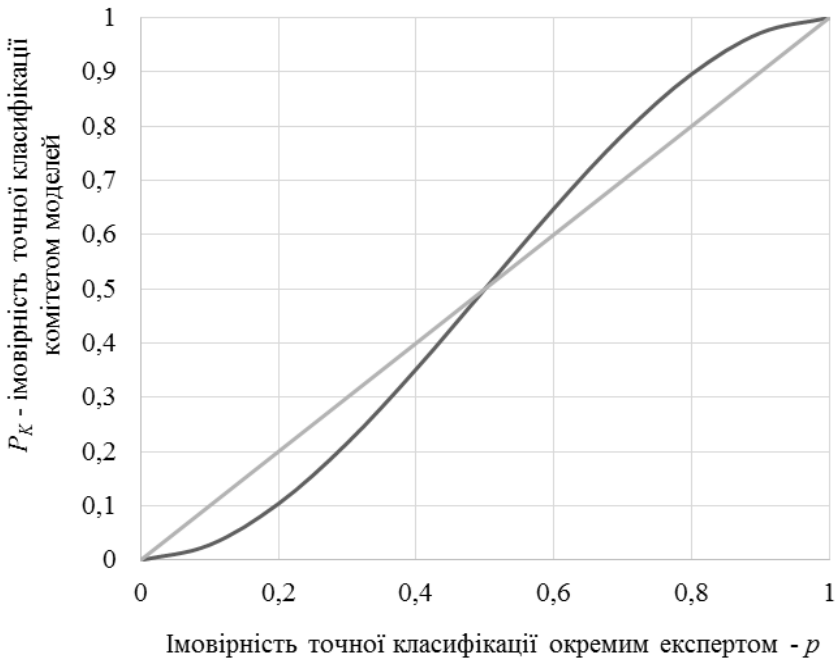
Рис. 4. Вигляд залежності ймовірності точної класифікації комітетом моделей P_K від точної класифікації окремим експертом p (побудовано з використанням [3])
